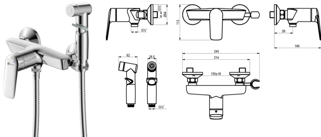
Смеситель с гигиеническим душем LM11418C
