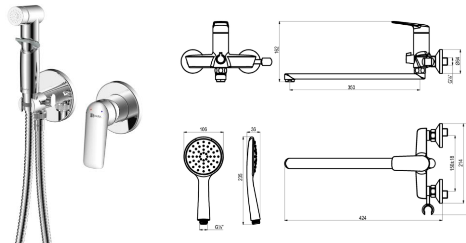
Смеситель с гигиеническим душем встраиваемый LM11419C
