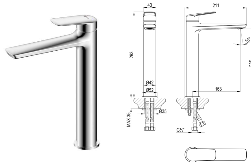
Смеситель для умывальника монолитный LM11409C
