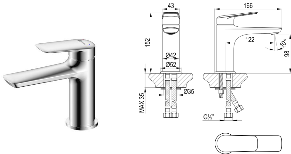
Смеситель для умывальника монолитный LM11406C
